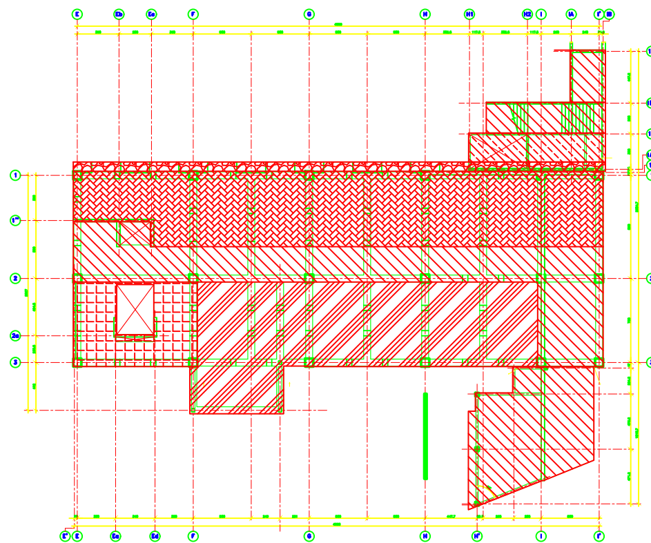
PLANTA CIELO PISO 1° ESCALA 1:150
