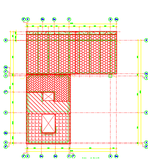
PLANTA CIELO 1° SUBTERRANEO ESCALA 1:150
