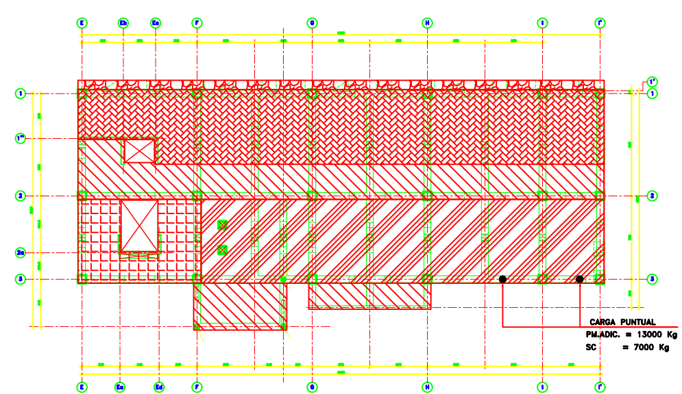
PLANTA CIELO PISO 2° ESCALA 1:150
